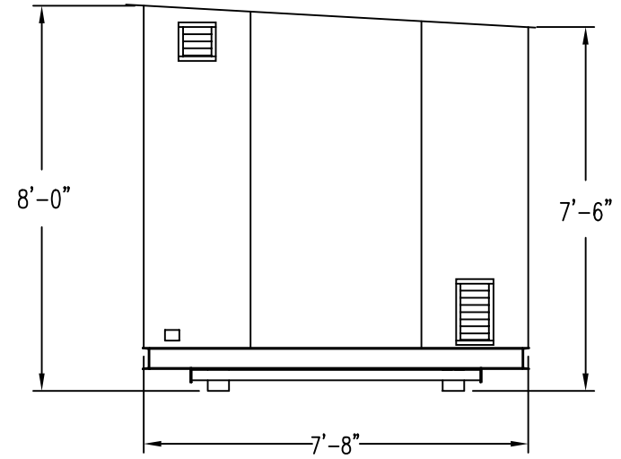
RIGHT ELEVATION
